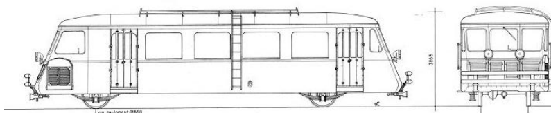
Autorail Billard type A-75-D n°901-903. c.f. de Mamers à Saint-Calais
